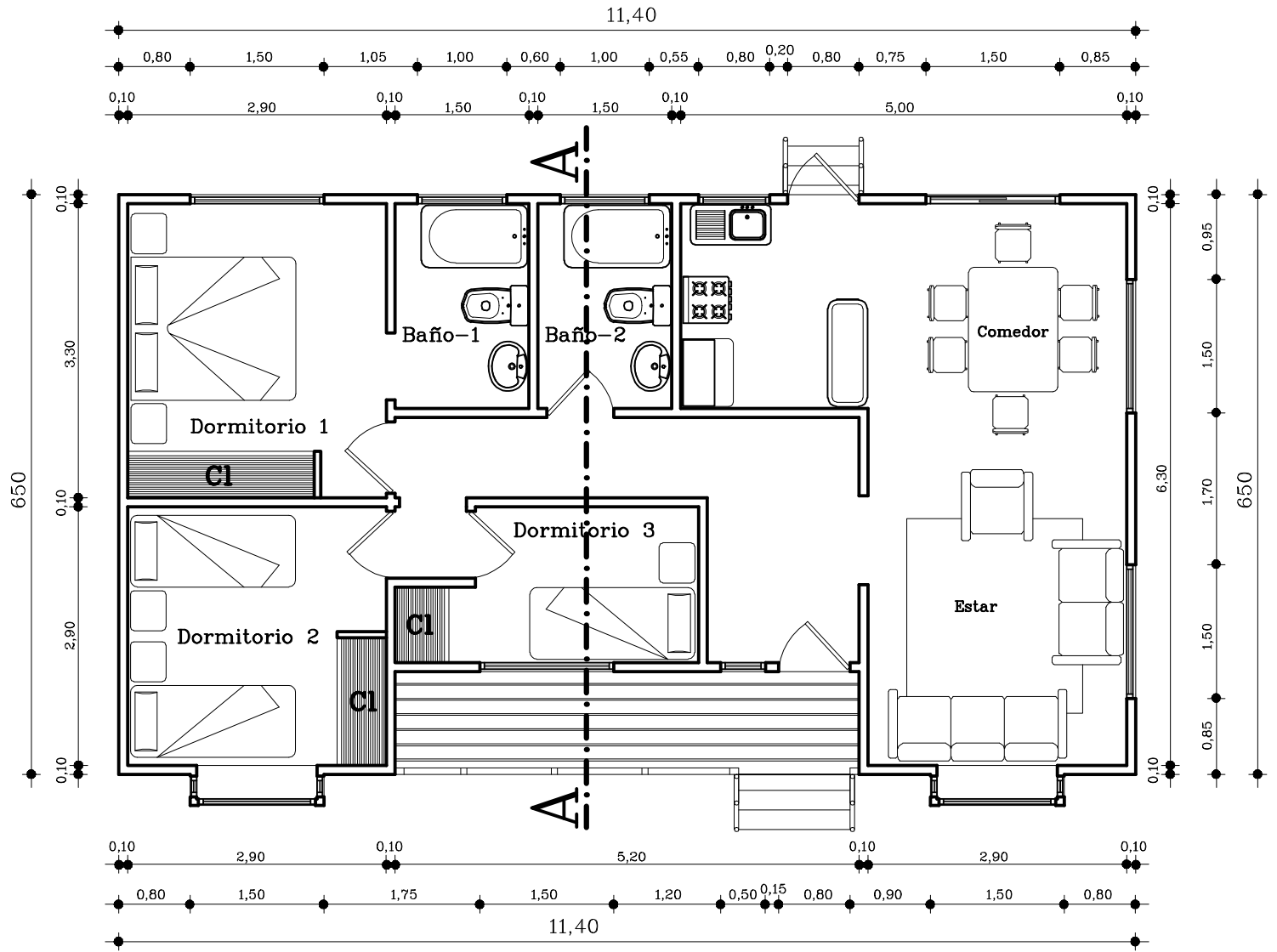
PLANTA GENERAL ESCALA 1:50
